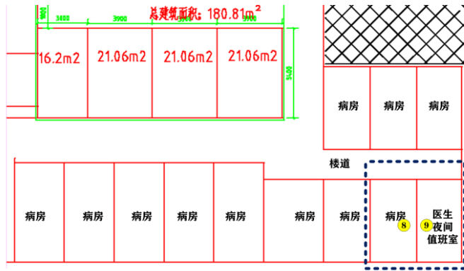
病房楼三层病房 局部平面
