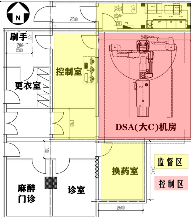
图 11-3 门诊楼 DSA（大 C）场所平面布局图示意图
