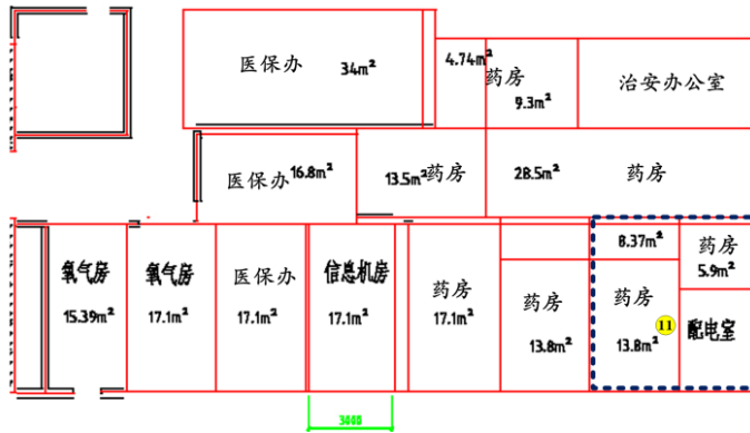
图 8-4 病房楼拟建中 C 机房场所及楼上和楼下检测点位示意图
