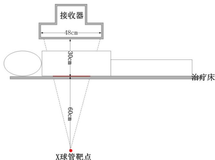
图 11-4 DSA 照射示意图
