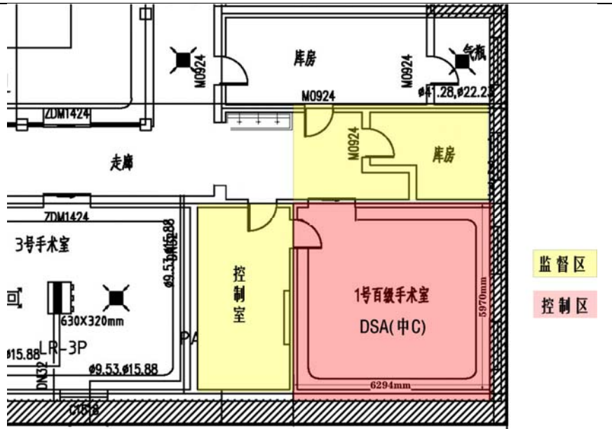
图 11-9 病房楼 1#手术室改建后平面布局图
