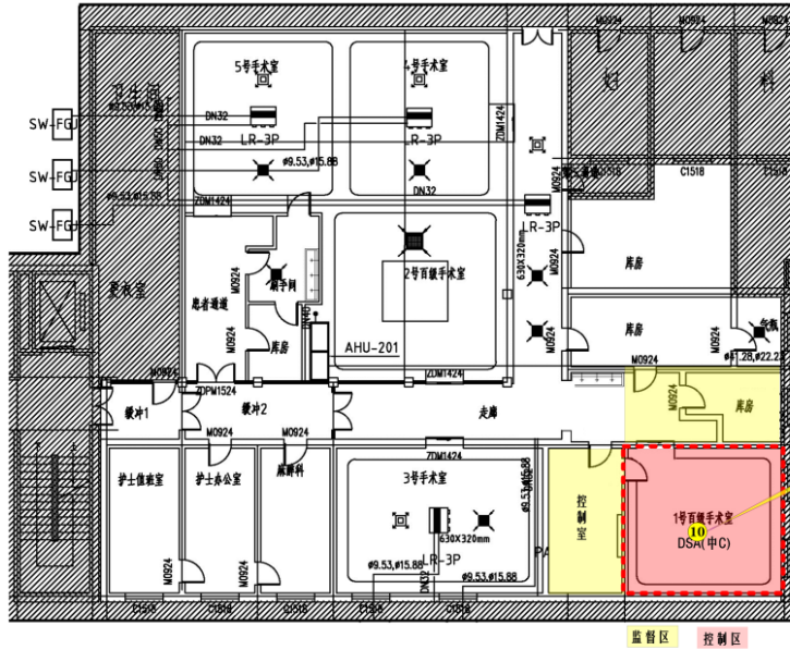
病房楼二层手术室 局部平面
