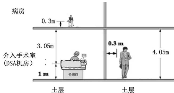
图 11-5 介入治疗手术室剖面示意图以及估算点位位置示意图
