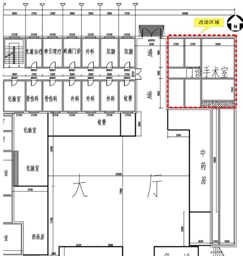
图 11-1 门诊手术室改造前平面布局示意图
