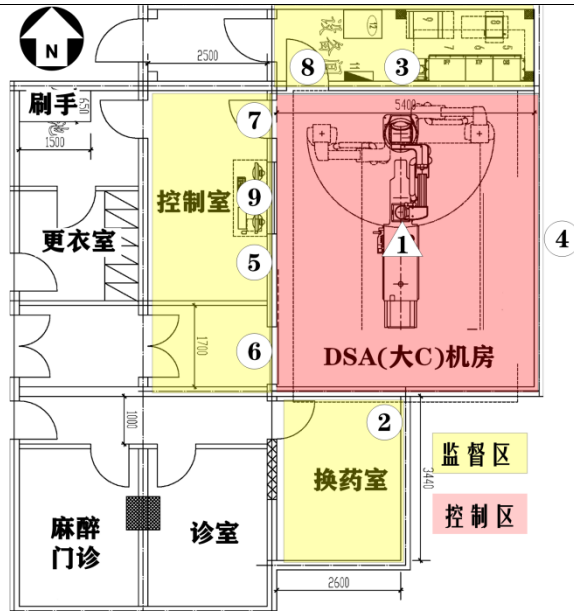
图 11-6 机房周围剂量估算点位置示意图
