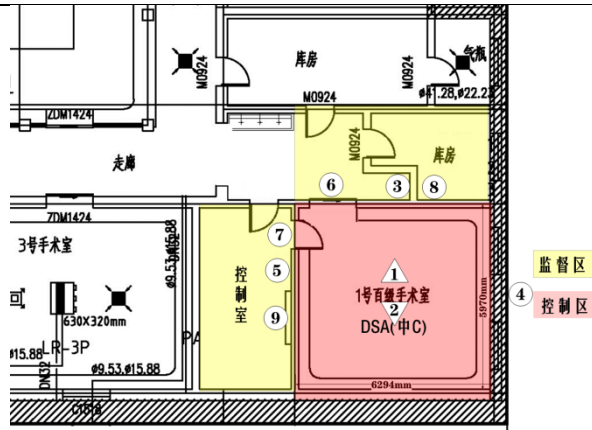
图 11-11 机房周围剂量估算点位置示意图
