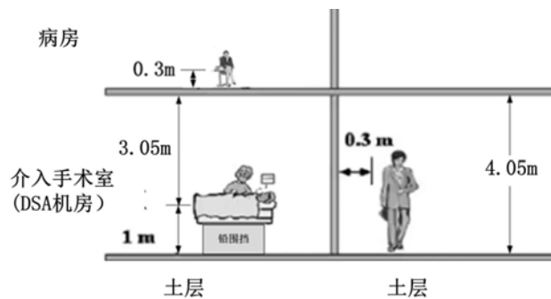
图 11-10 介入治疗手术室剖面示意图以及估算点位位置示意图
