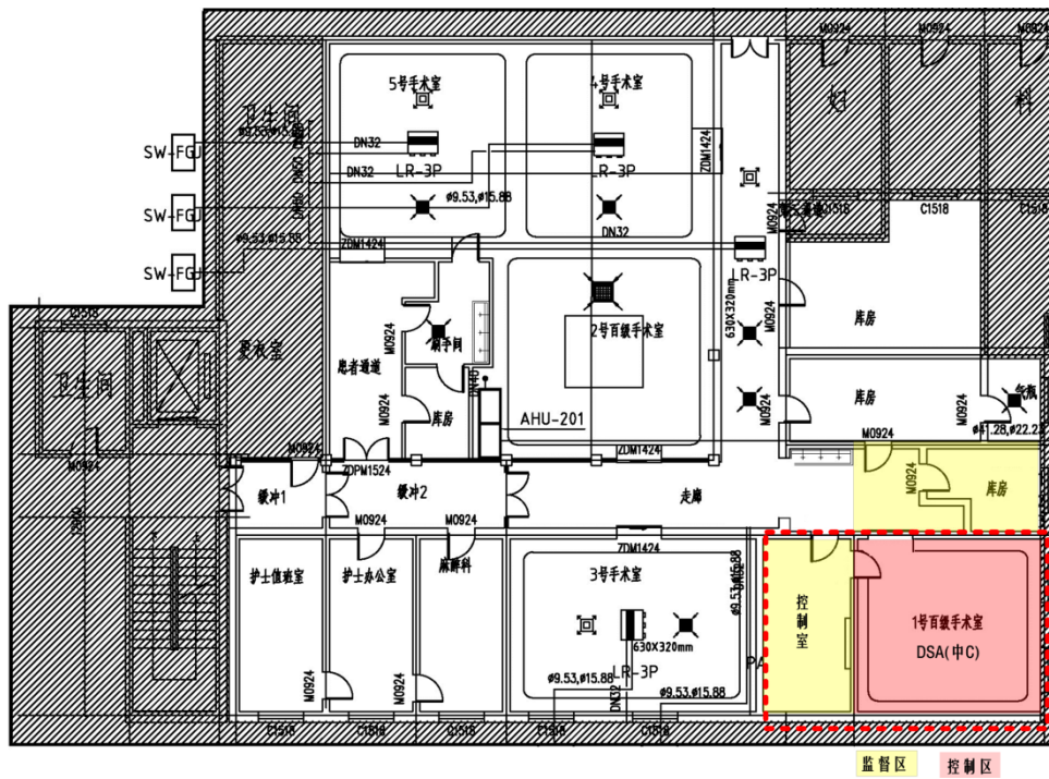
图 11-8 场所改建后 DSA 机房（中 C）平面布局示意图
